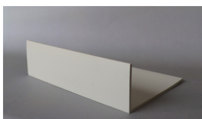
Cornière 60 x 25 x 1,5 mm
