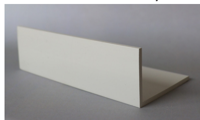
Cornière 100 x 60 x 2,2 mm
